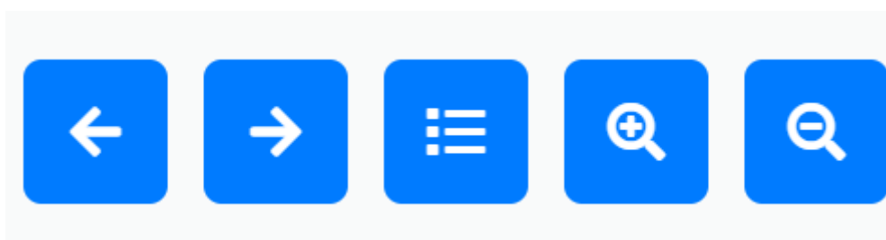
Рисунок 1 – Навигационное меню
